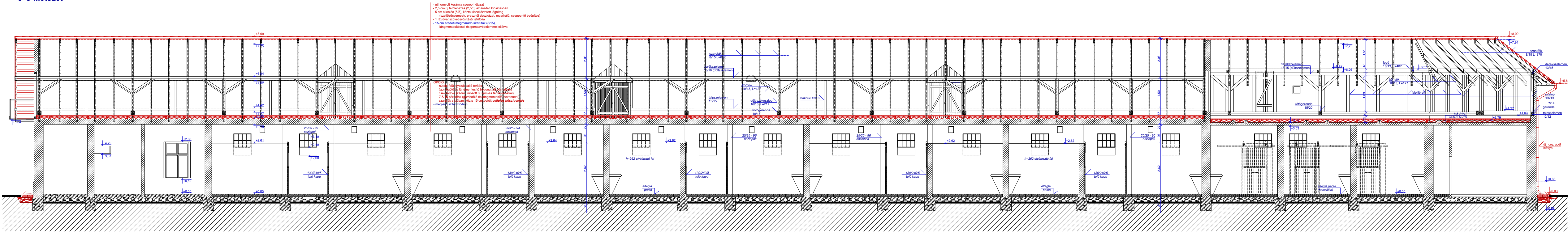
C-C Metszet
