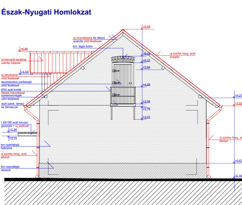
Észak-Nyugati Homlokzat
