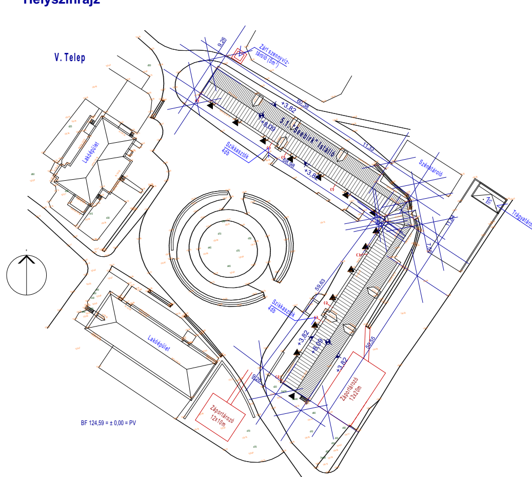
Helyszínrajz
