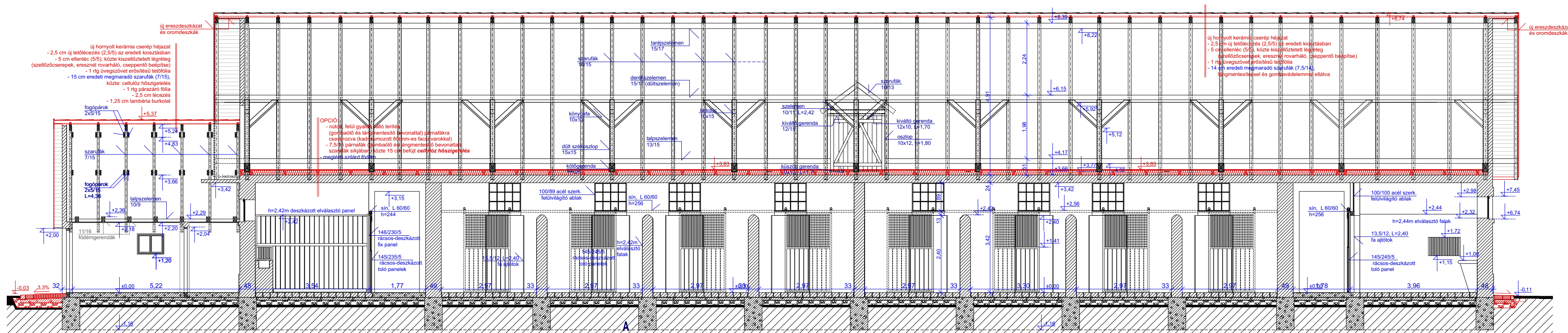
B-B Metszet
