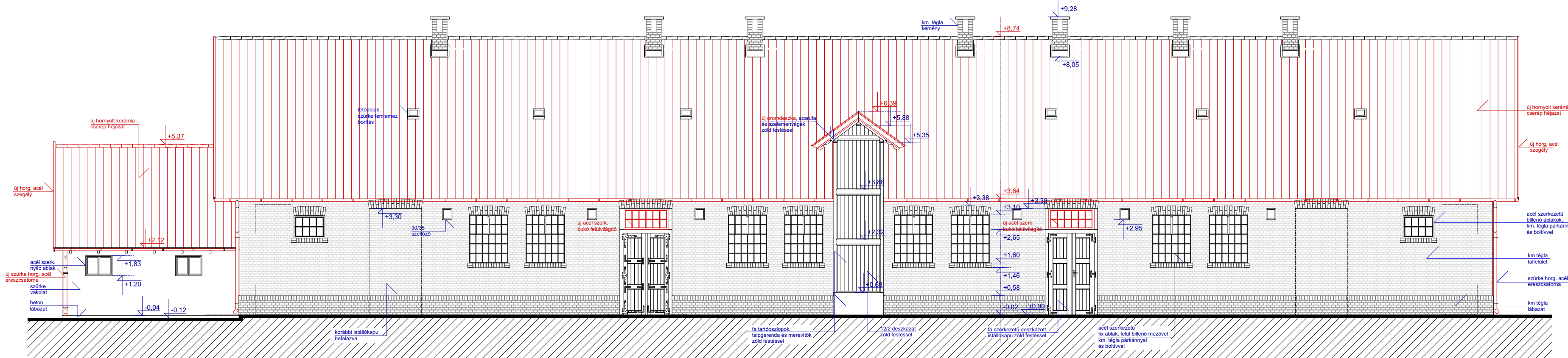
Észak-Keleti Homlokzat
