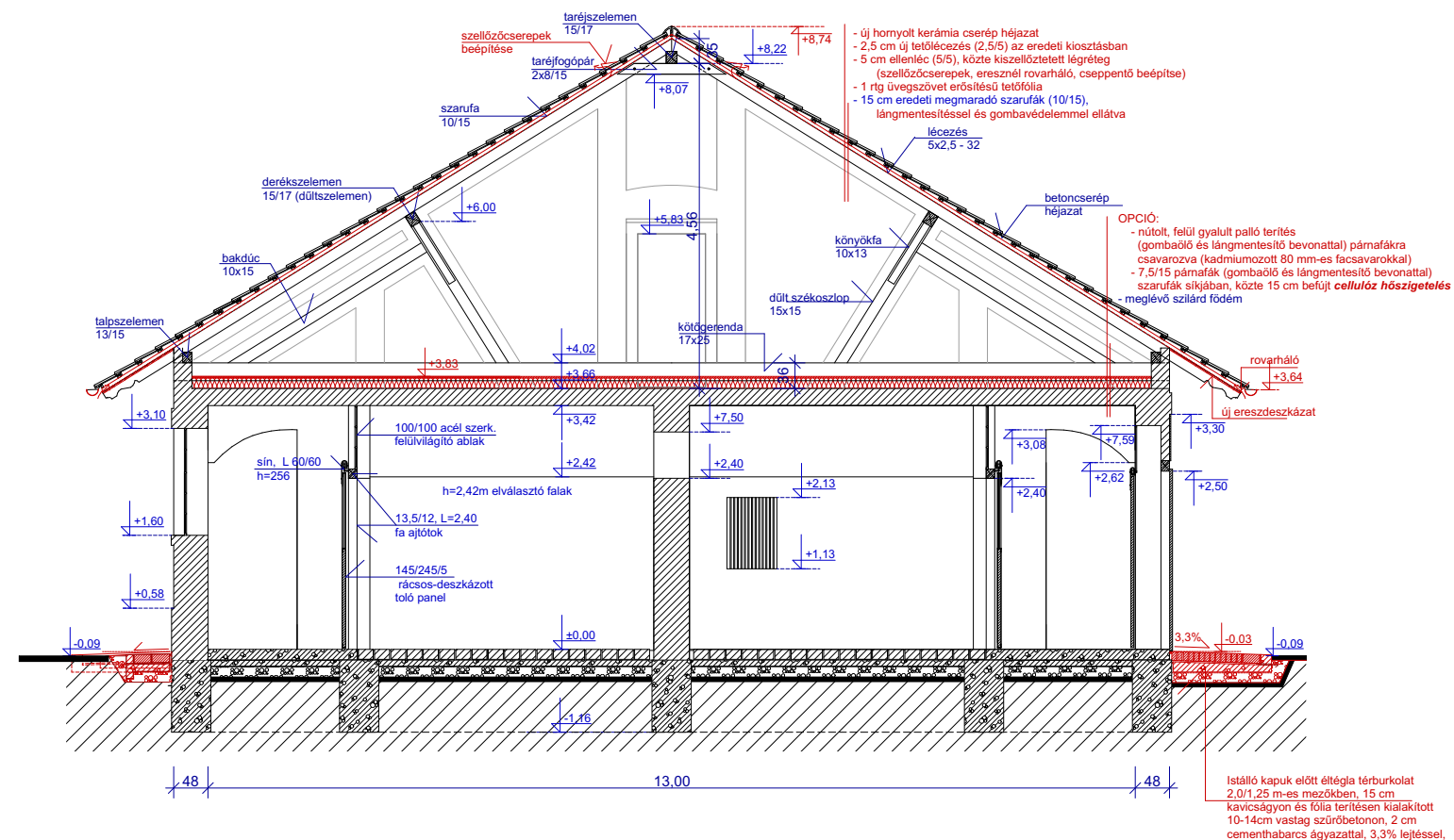
A-A Metszet
