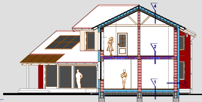
A-A Metszet
