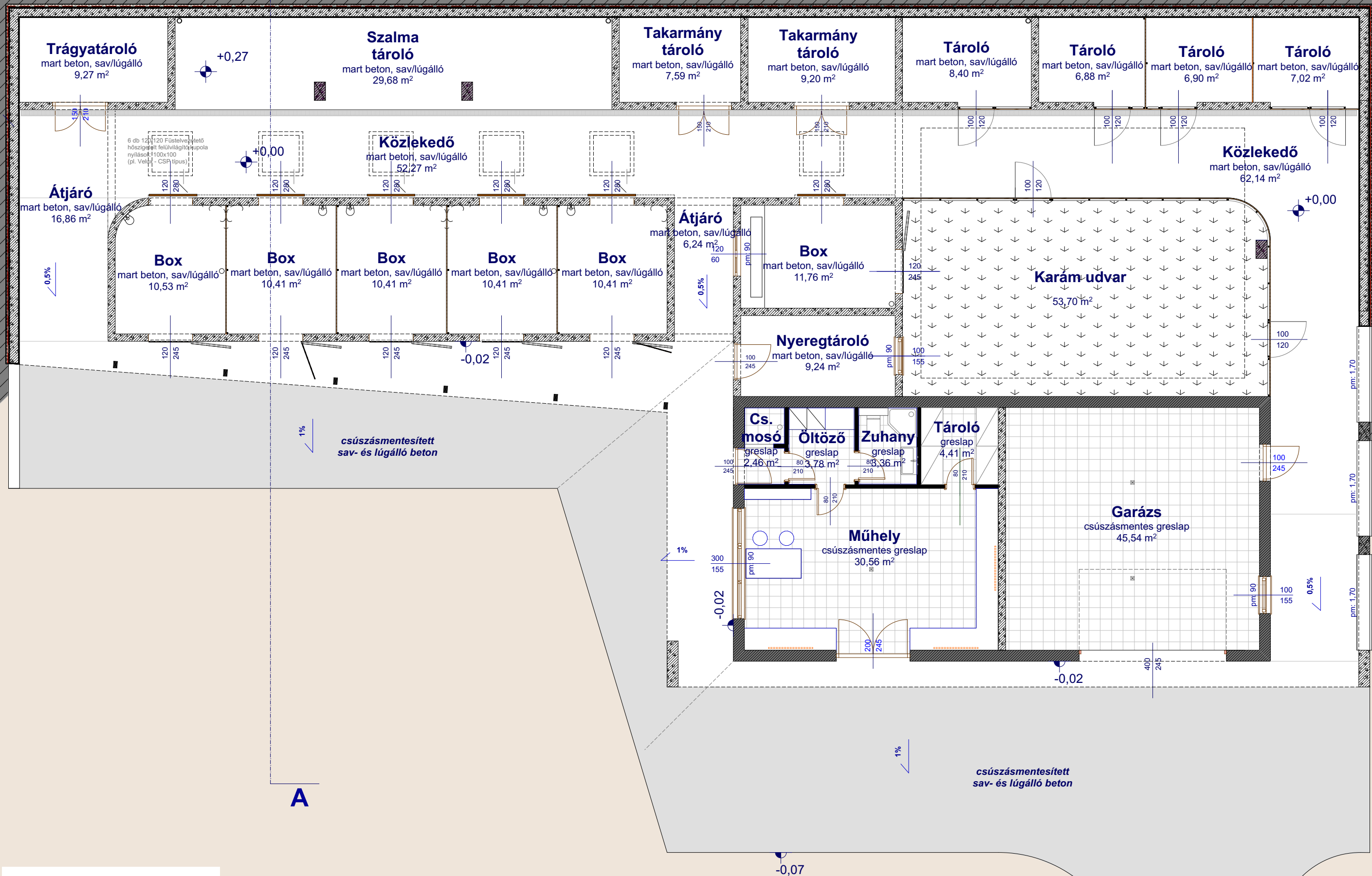
ALAPRAJZ
