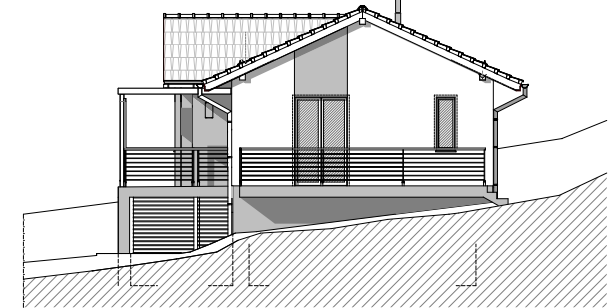
Észak-nyugati Homlokzat
