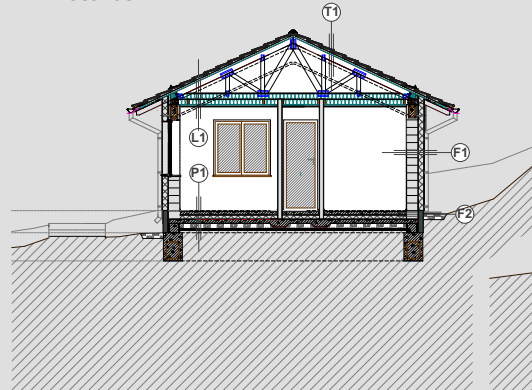
A-A Metszet
