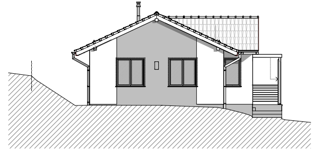
Észak-nyugati Homlokzat
