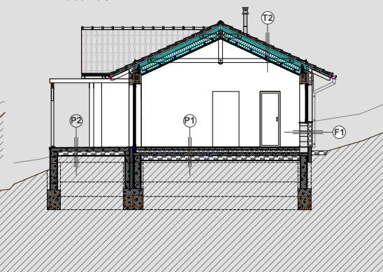
B-B Metszet
