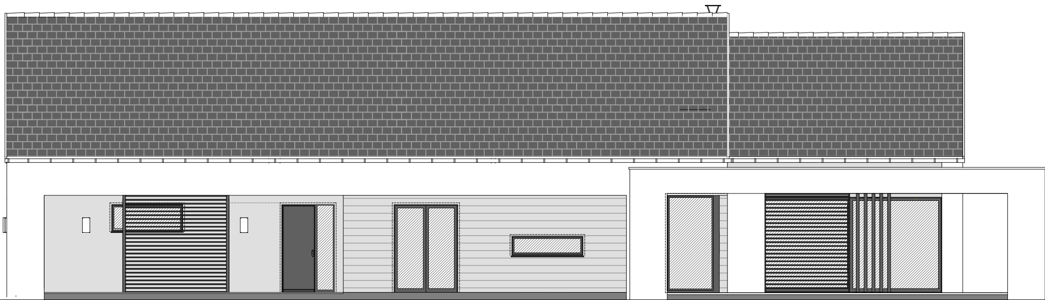
ÉSZAK-NYUGATI HOMLOKZAT
