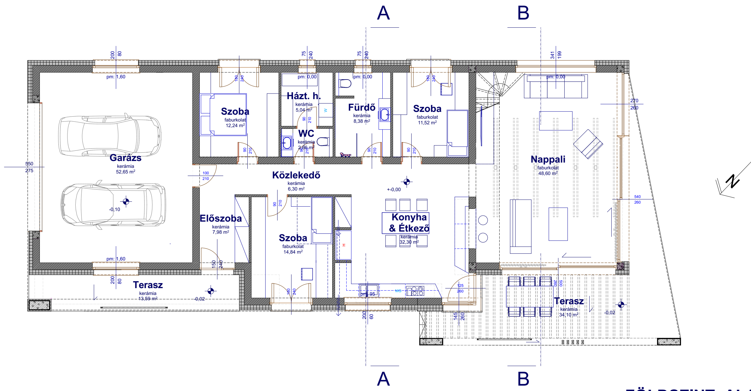
FÖLDSZINT ALAPRAJZ
