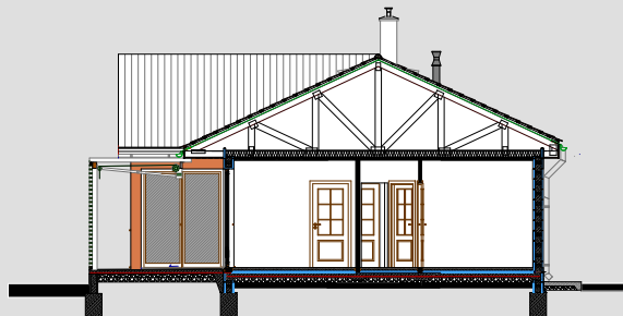
A-A Metszet
