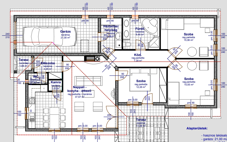
Alaprajz
