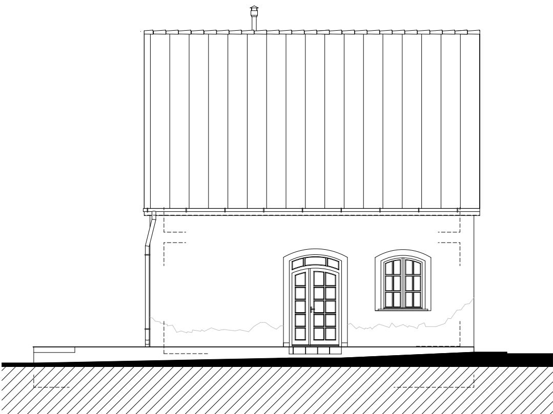
Keleti homlokzat (eredeti)
