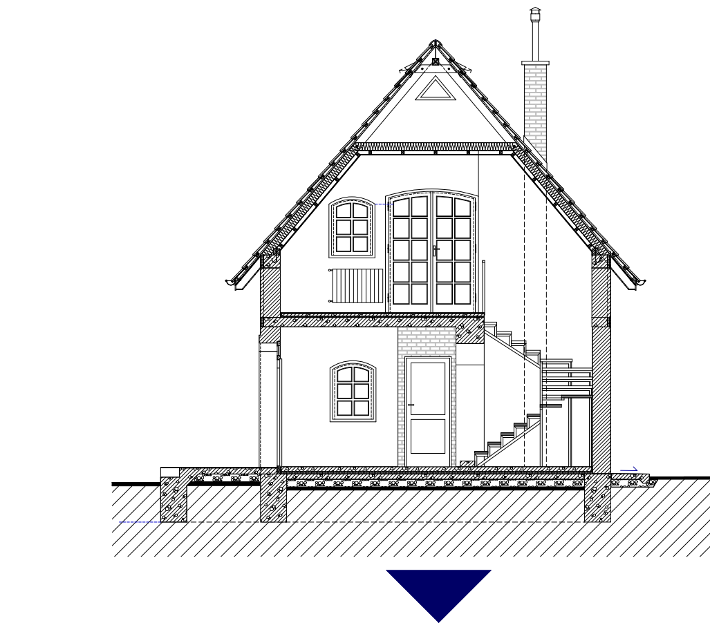
A-A metszet (tervezett)
