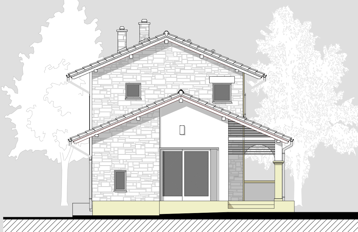
Déli homlokzat (tervezett)
