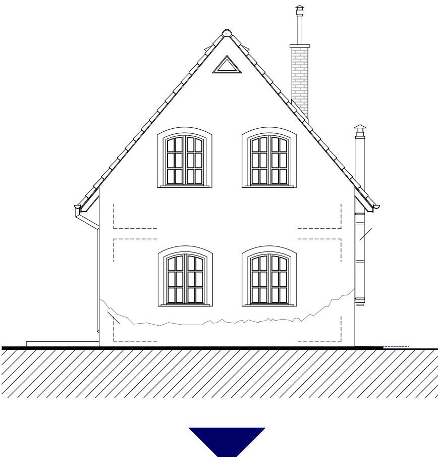
Északi (utcai) homlokzat (tervezett)
